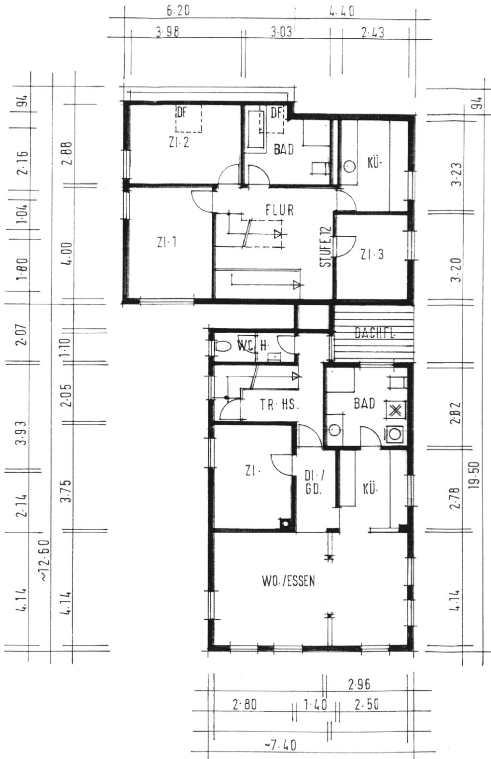
GH.846 – Grundriss OG
